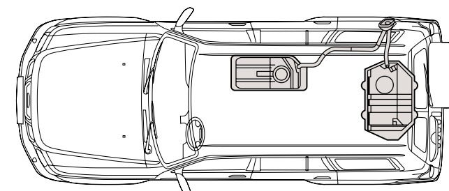
مكان خزان الوقود الإضافي Sub-fuel tank location
